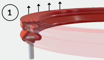
Axiale Erweiterung Axial Expansion Expansión Axial
