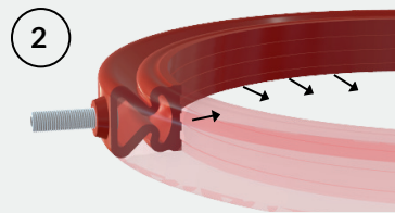
Innere Radiale Erweiterung Internal Radial Expansion Expansión Radial Interna
